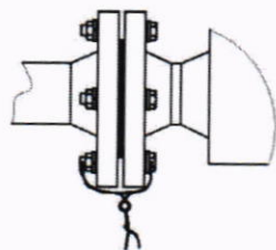
Рисунок А.1 – Схема пломбировки фланцев счетчиков – расходомеров массовых.
