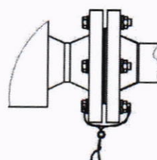
Рисунок А.1 – Схема пломбировки фланцев счетчиков – расходомеров массовых.
