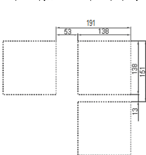
Рисунок 1а- Разметка щита для прибора исполнения IP20
