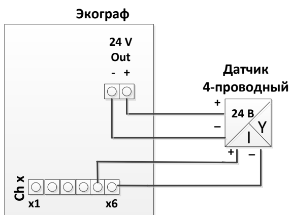
Рисунок 8 – Подключение 4-проводного датчика
