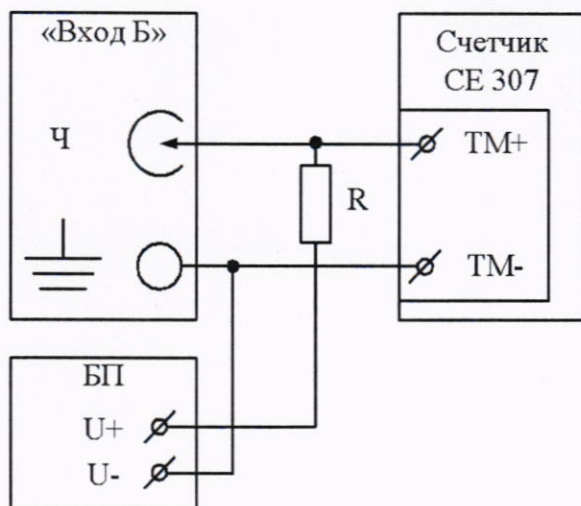
Рисунок 9.2 - Схема соединения для проверки точности часов
