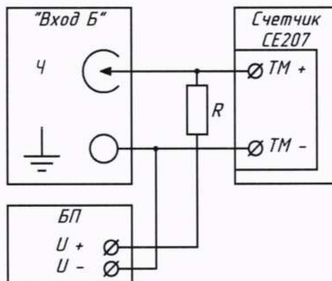
Рисунок 9.1 - Схема соединения для определения погрешности хода часов счетчика с электронным испытательным выходом
