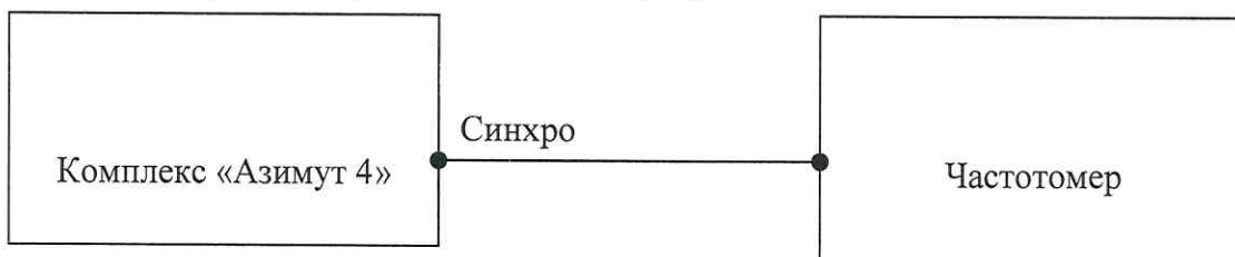
Рисунок 8 – Схема для определения погрешности следования кадровых синхроимпульсов
