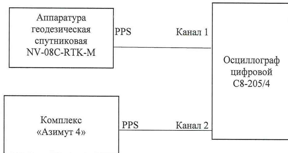
Рисунок 12 – Схема выполнения измерений
