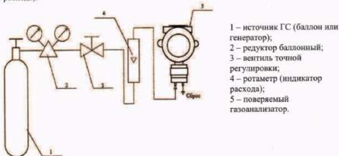
Рисунок 1 - Схема подачи ГСО-ПГС на вход газоанализатора при проведении поверки
