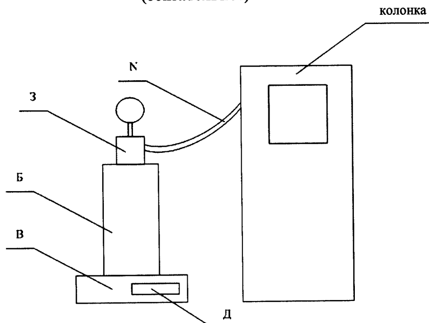
Рисунок Б.1 – Схема подключения колонки при проведении поверки
