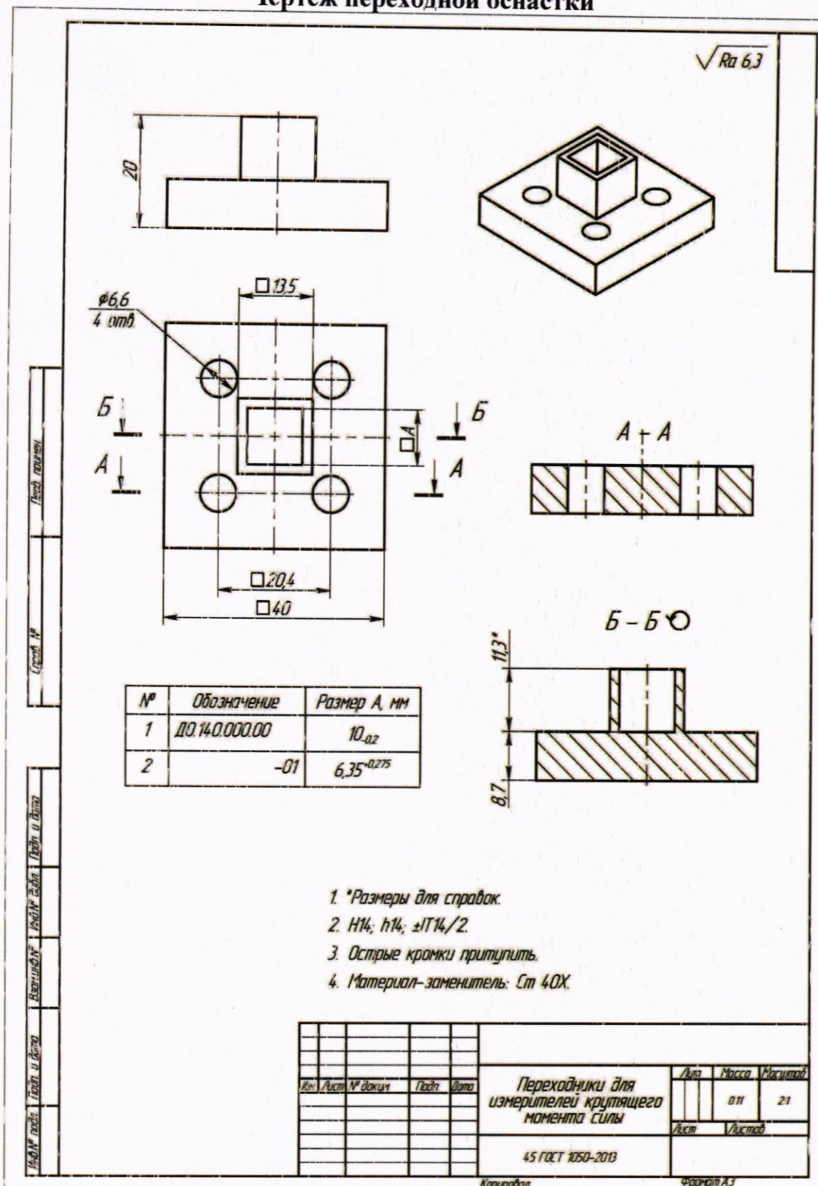
Рисунок Б.1 – Чертёж переходной оснастки
