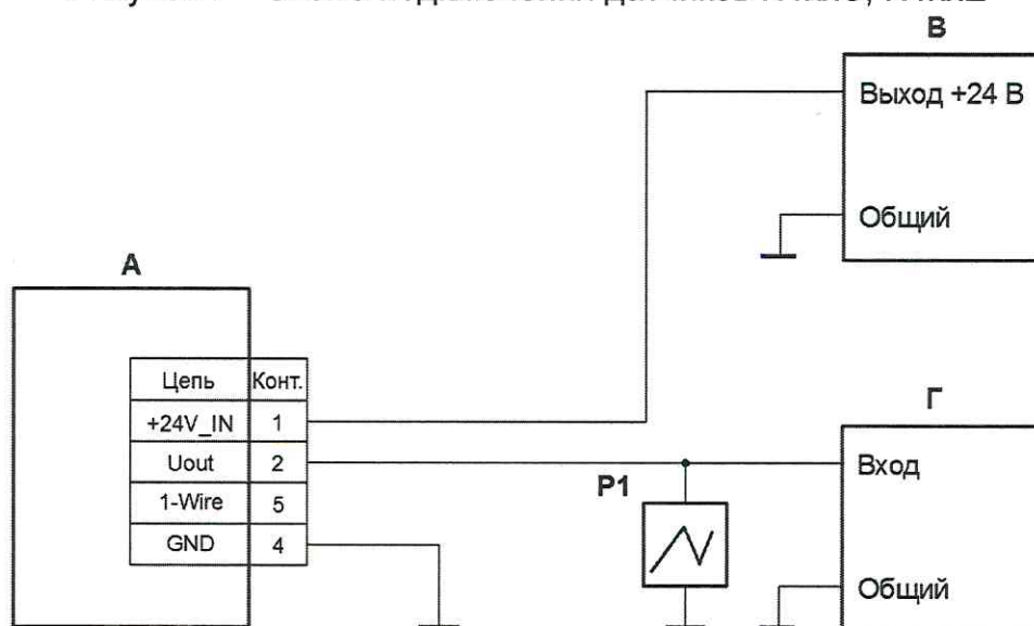
Рисунок 1 – Схема подключения датчиков N1xxC, N1xxE
