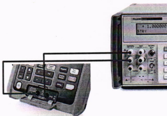
Рисунок 3 – Схема соединения приборов при определении погрешности измерения напряжения постоянного и переменного тока, электрического сопротивления постоянному току, электрической емкости
