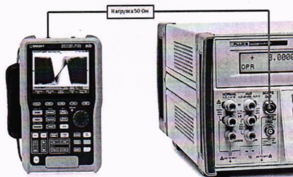
Рисунок 2 – Схема соединения приборов при определении времени нарастания переходной характеристики и определении относительной погрешности частоты внутреннего опорного генератора.
