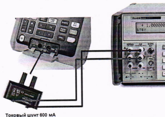
Рисунок 4 – Схема соединения приборов при определении погрешности измерения силы постоянного и переменного тока на пределах 60 и 600 мА
