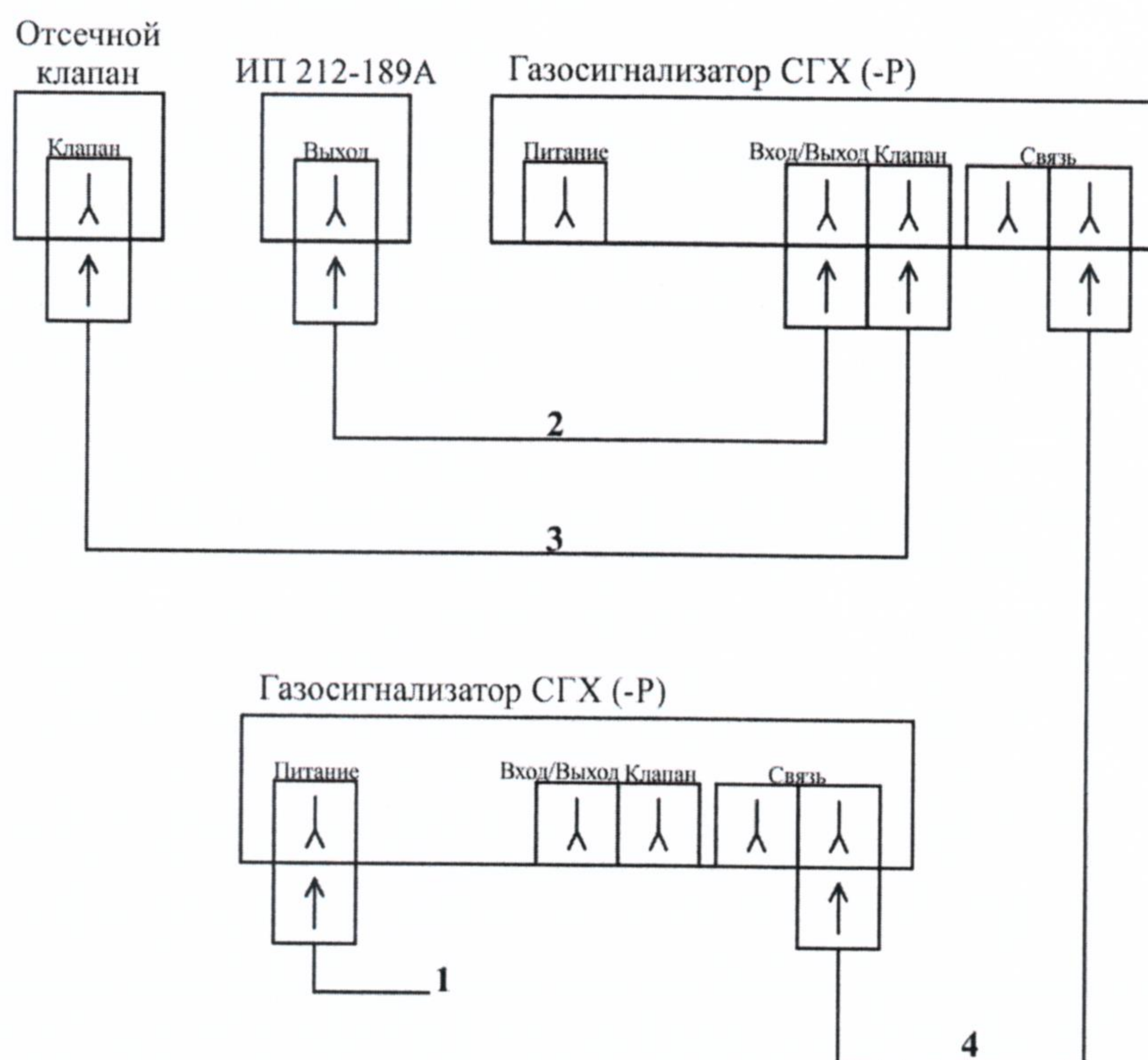
Рис. Б2 Пример схемы подключения газосигнализаторов СГХ. На рисунке отображены: •1 – подключение источника питания; •2 – подключение газосигнализатора и отсечного клапана; •3 – подключение газосигнализаторов.
