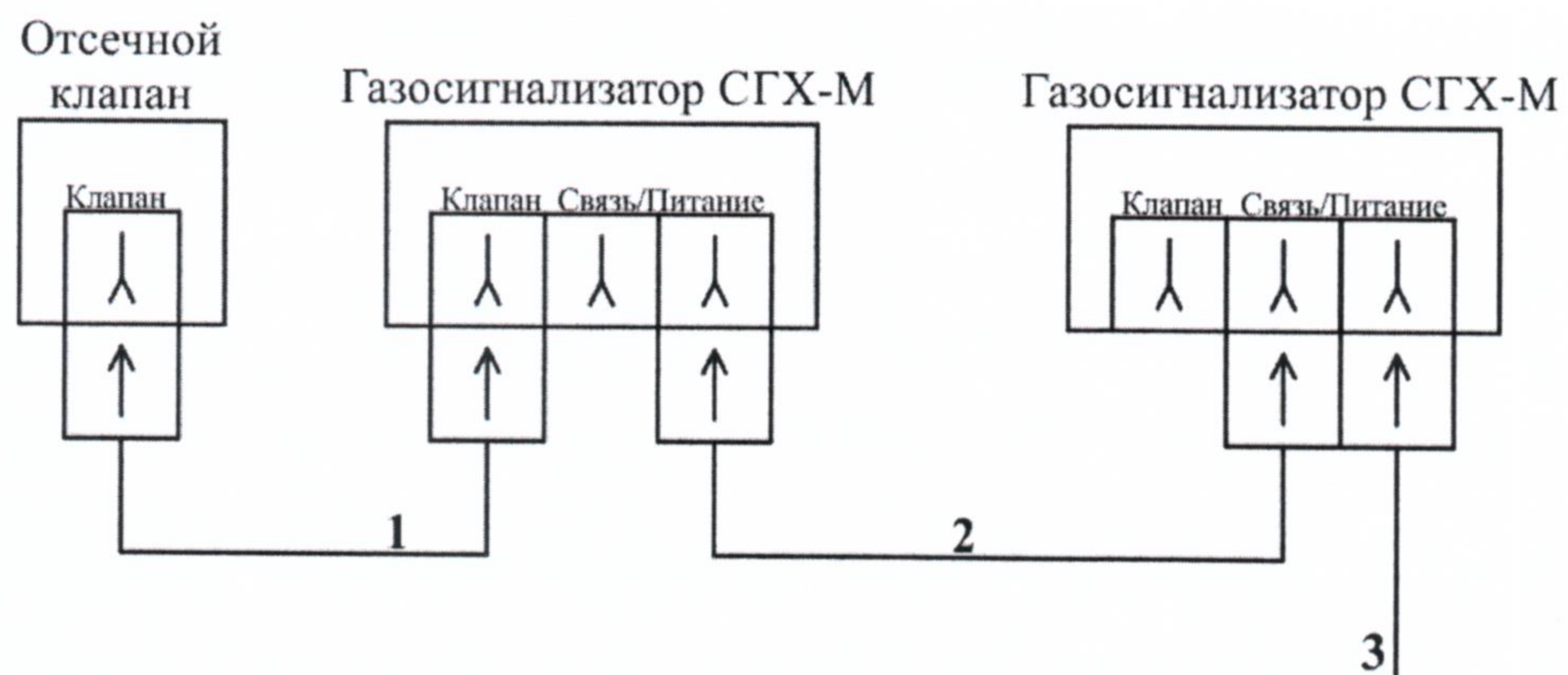
Рис. Б3 Пример схемы подключения газосигнализаторов СГХ-М. На рисунке отображены:
