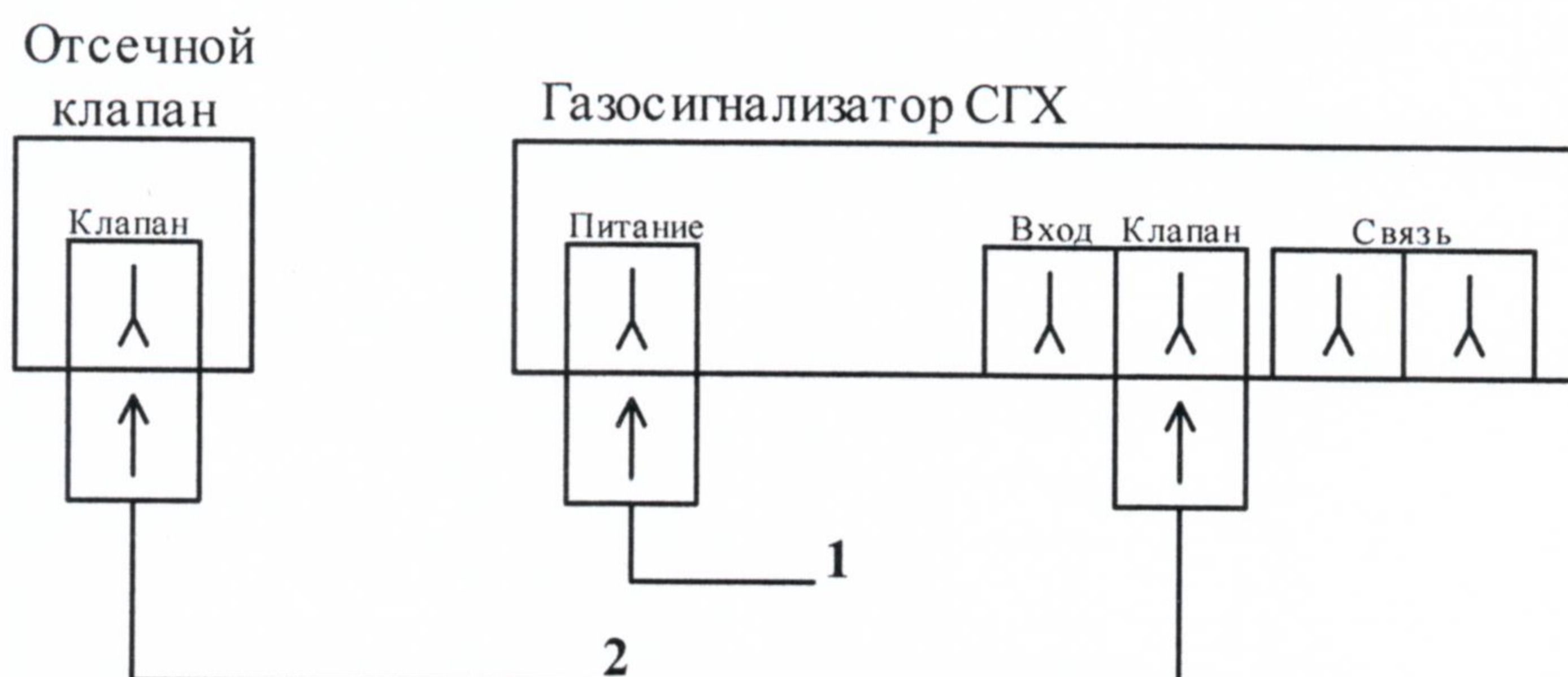
Рис. Б1 Пример схемы подключения газосигнализатора СГХ к клапану. На рисунке отображены: •1 – подключение источника питания; •2 – подключение сигнализатора и отсечного клапана.
