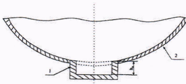
1 – прямик; 2 – цилиндрическая часть танка h_я – высота прямика
