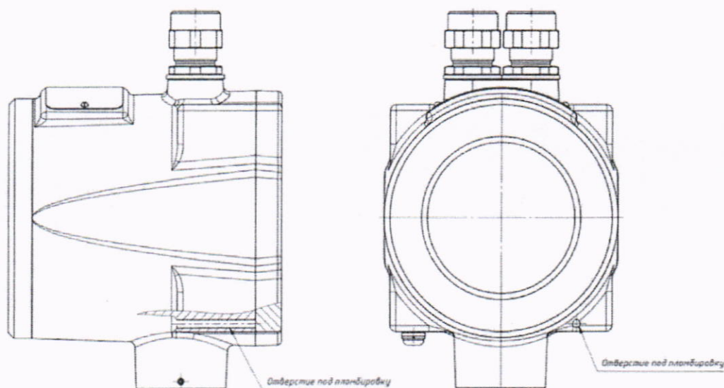
Р и с у н о к А.1 – Пример схемы и обозначения мест пломбировки с нанесением знака поверки на массовые расходомеры НАРА
