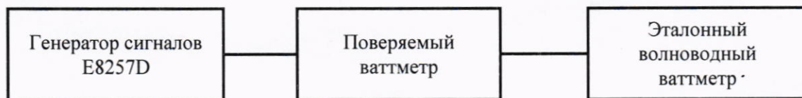
Рисунок 3 – Схема измерений для определения относительной погрешности измерений мощности
