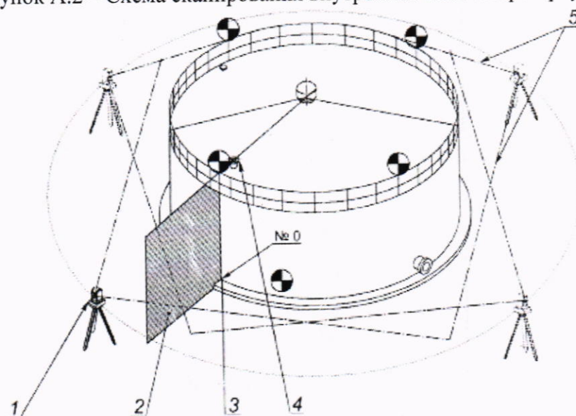
1 - станция сканирования; 2 - плоскость A; 3 - сферическая марка, установленная на ограждении кровли; 4 - точка измерения базовой высоты; 5 - сектор сканирования; сферическая марка
