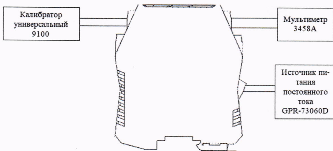
Рисунок 3 – Схема подключения для определения приведенной (к верхнему пределу диапазона выходного сигнала) основной погрешности преобразований входных сигналов напряжения постоянного и переменного тока, силы переменного тока и входного сигнала от преобразователей термоэлектрических по ГОСТ Р 8.585-2001 в выходной сигнал
