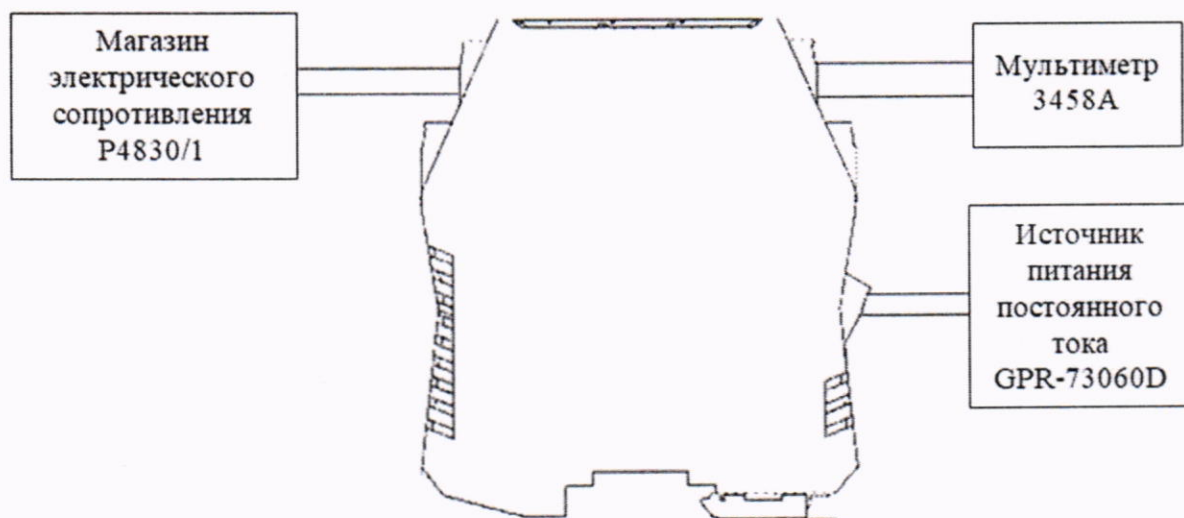
Рисунок 2 – Схема подключения для определения приведенной (к верхнему пределу диапазона выходного сигнала) основной погрешности преобразований входного сигнала сопротивления постоянному току и входного сигнала от термопреобразователей сопротивления в выходной сигнал
