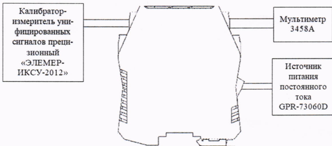
Рисунок 1 – Схема подключения для определения приведенной (к верхнему пределу диапазона выходного сигнала) основной погрешности преобразований входного сигнала силы постоянного тока в выходной сигнал
