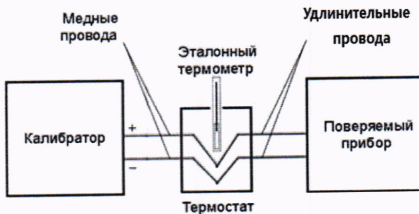
Рисунок 1 – Схема подключения
