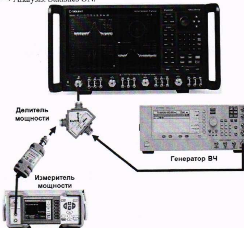
Рисунок 3 – Схема соединения приборов для определения абсолютной погрешности измерений уровня мощности
