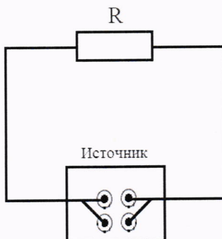
Рисунок 3.1 – Схема подключений для определения абсолютной основной погрешности измерений электрического сопротивления постоянному току (для значения сопротивления постоянному току 2 Ом необходимо соединить последовательно катушку P321 и меру P3030)
