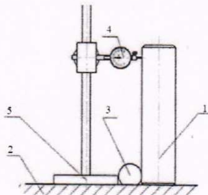
Рисунок 3 – Схема определения отклонения наружной измерительной поверхности угольника к опорной определяют методом сличения с эталонным угольником
