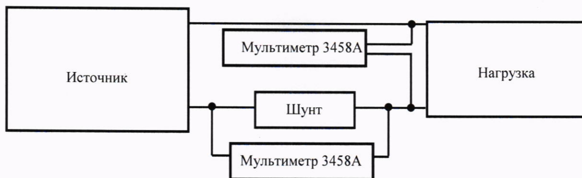
Рисунок 3 - Структурная схема определения абсолютной погрешности установки электрического сопротивления, электрической мощности постоянного тока
