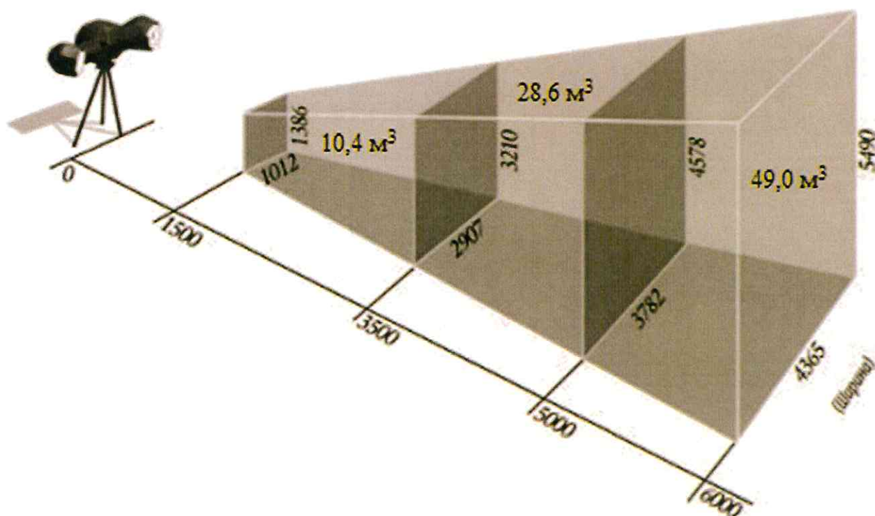
Рисунок А.2 – Схема измерительных объёмов модификации AM.TECH TrackScan Sharp 49
