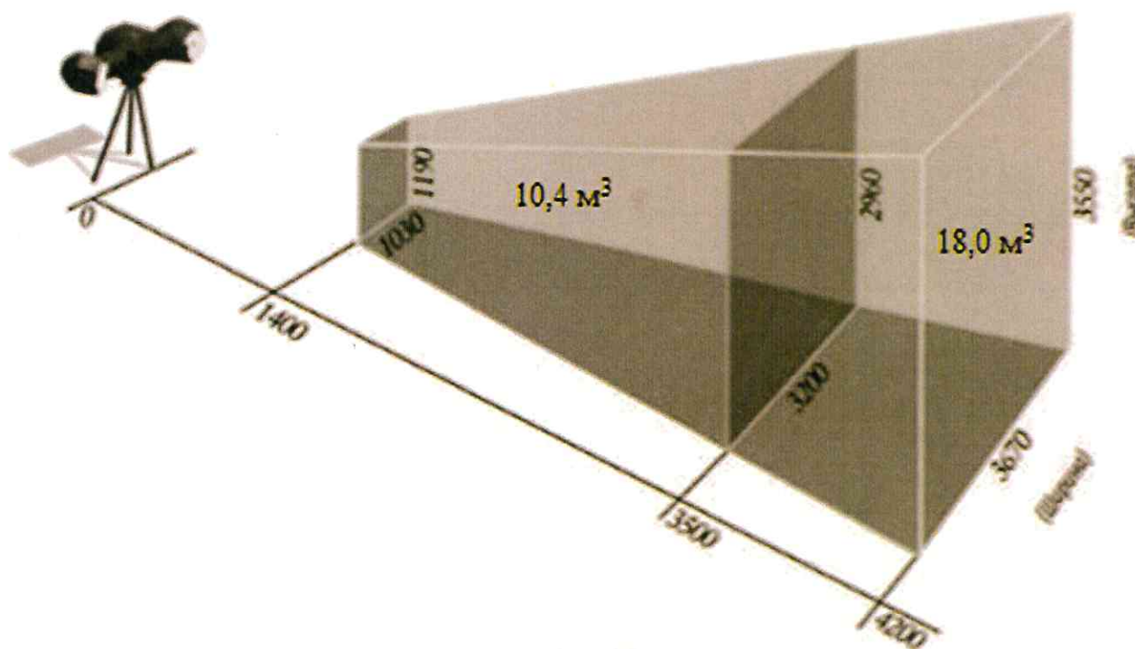
Рисунок А.1 – Схема измерительных объёмов модификаций AM.TECH TrackScan P542 / AM.TECH TrackScan P550
