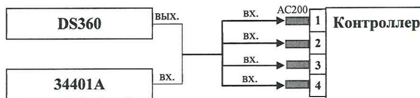
Рисунок 16 – Схема подключения
