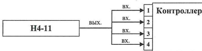
Рисунок 11 – Схема подключения
