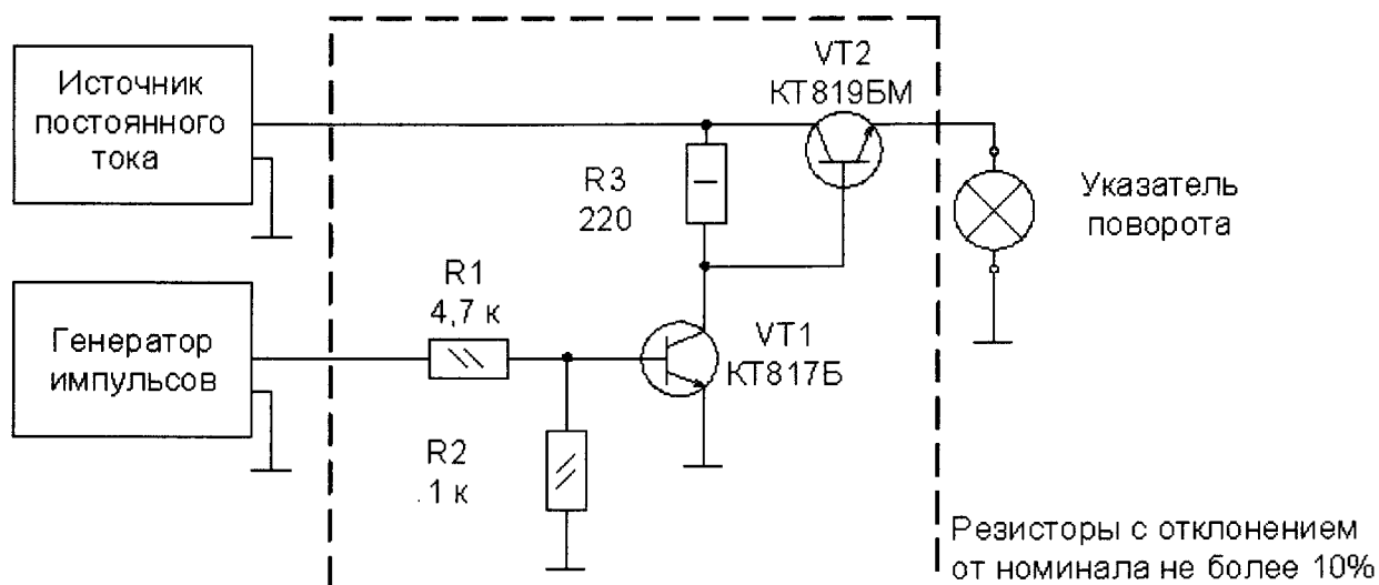
Рисунок 2 – Схема подключения указателя поворота
