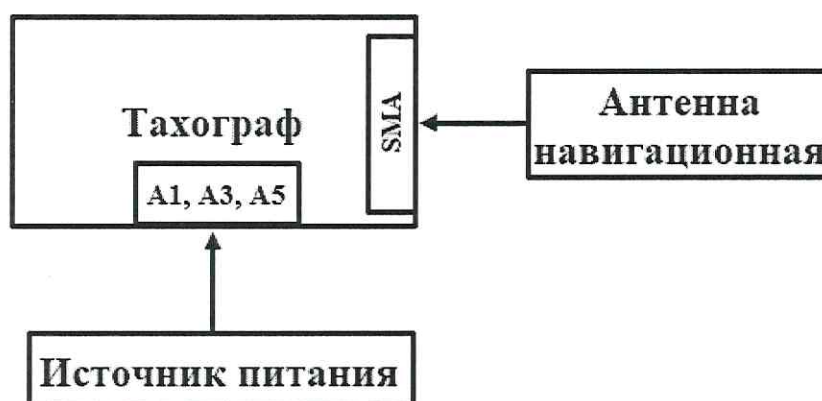
Рисунок 1 – Схема проведения измерений при опробовании
