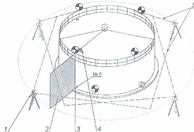
1 - станция сканирования; 2 - плоскость А; 3 - сферическая марка, установленная на ограждении кровли; 4 - точка измерения базовой высоты; 5 - сектор сканирования; сферическая марка
