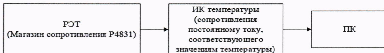
Рисунок 4 - Схема поверки ИК температуры (сопротивления постоянному току, соответствующего значениям температуры), РЭТ магазин сопротивления Р4831
