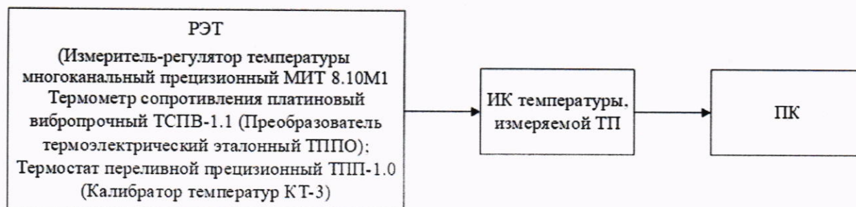
Рисунок 5 - Схема поверки ИК температуры, измеряемой КТХА (К), РЭТ МИТ 8.10М1 с ТСПВ-1.1 (ТППО) и ТПП-1.0 (КТ-3)
