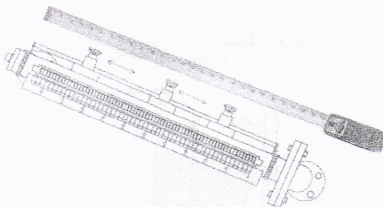
Рисунок 3 – Поверка уровнемера с помощью измерительной рулетки в лабораторных условиях
