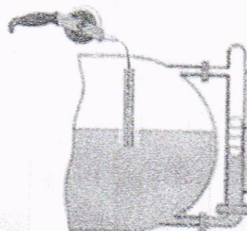
Рисунок 2 – Поверка уровнемера без демонтажа с помощью измерительной рулетки с грузом
