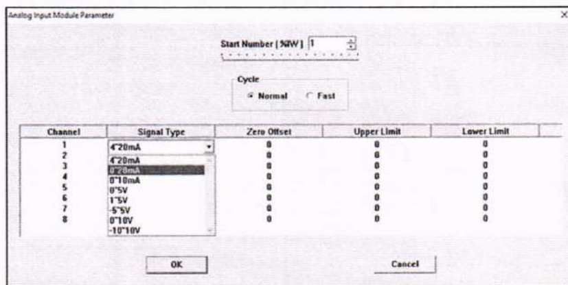
Рисунок 6 – Параметры преобразователей
