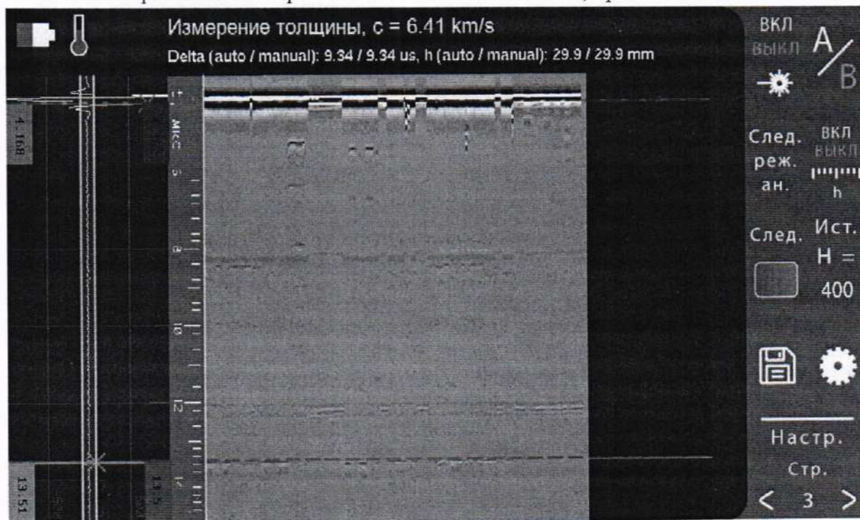
Рисунок 2 – Отображение донного сигнала на А и В-скане
