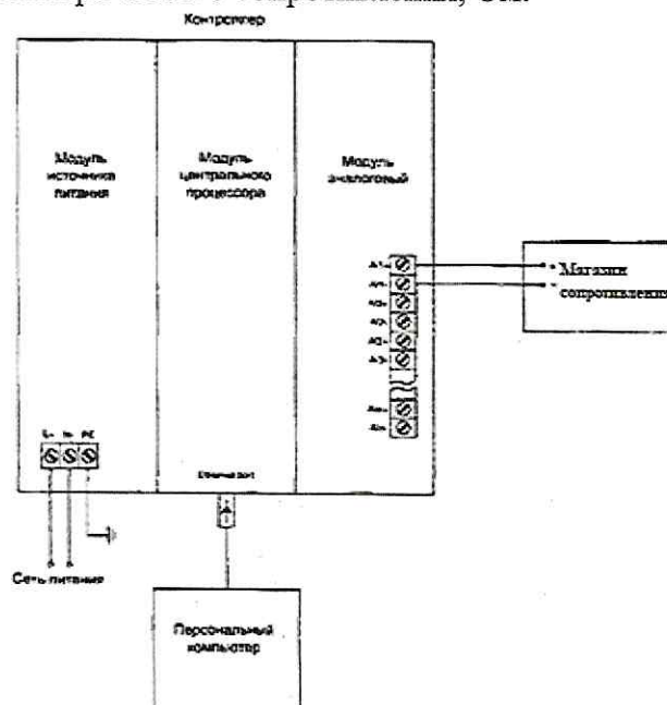
Рисунок 3 – Схема определения погрешности измерений сигналов электрического
