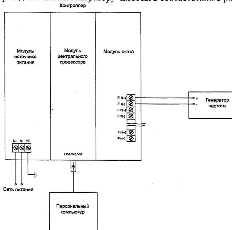
Рисунок 4 – Схема определения погрешности измерений частотных сигналов
