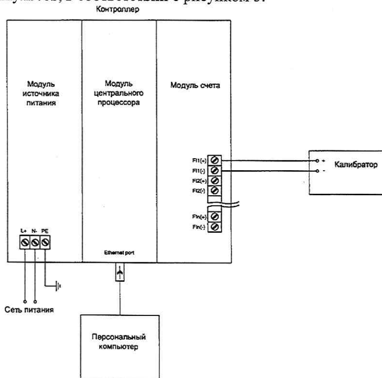
Рисунок 5 – Схема определения погрешности измерений импульсных сигналов
