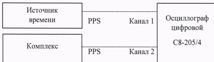
Рисунок 1 – Схема выполнения измерений
