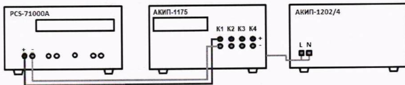
Рисунок 2 – Схема соединения приборов при определении абсолютной погрешности воспроизведения силы постоянного тока
