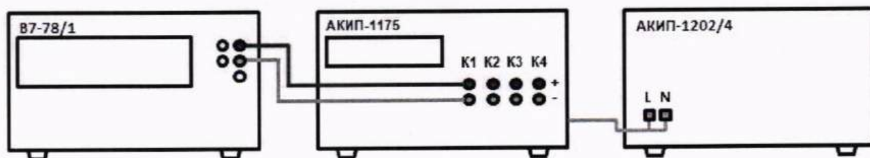
Рисунок 1 – Схема соединения приборов при определении абсолютной погрешности воспроизведения напряжения постоянного тока
