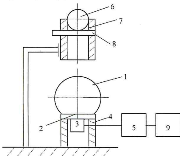
Рисунок 1 – Схема проверки частоты установочного резонанса
