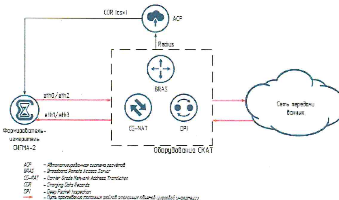
Рисунок 1 – Схема поверки СИПД
