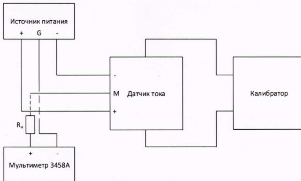
Рисунок 1 – Схема подключения (R н – сопротивление нагрузки, 1 кОм)
