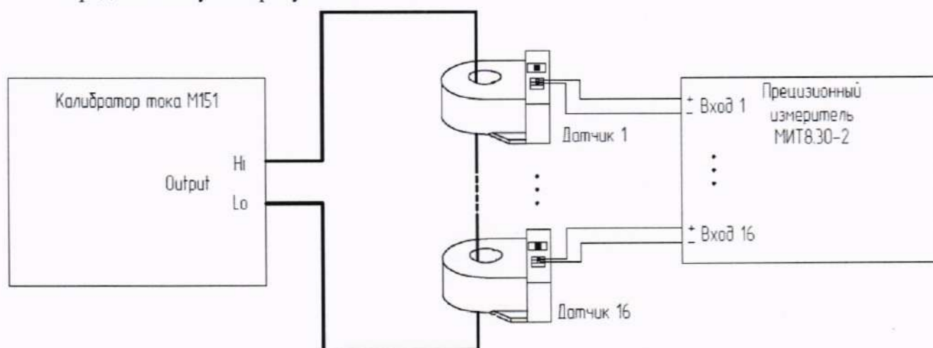
Рисунок.1 — Схема подключения оборудования и датчиков с диапазонами до 100 А при питании от встроенного источника питания МИТ8.30-2
