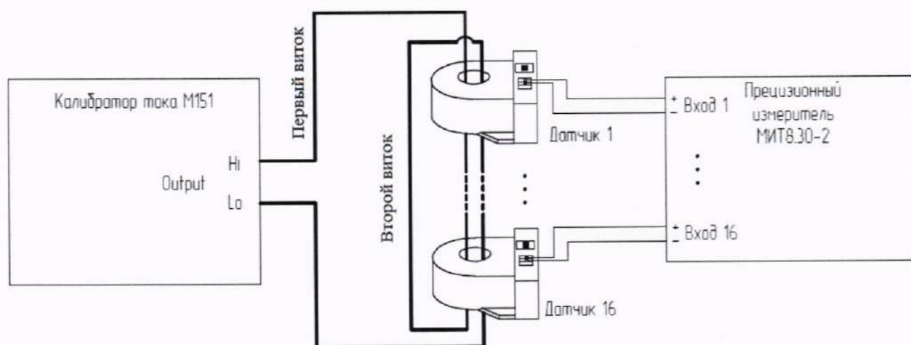
Рисунок.2 — Схема подключения оборудования и датчиков с диапазонами от 100 А при питании от встроенного источника питания МИТ8.30-2
