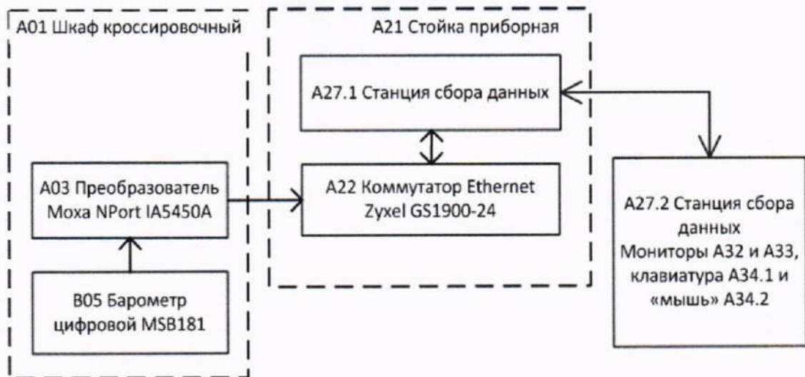
Рисунок 20 – Схема ИК давления атмосферного воздуха
