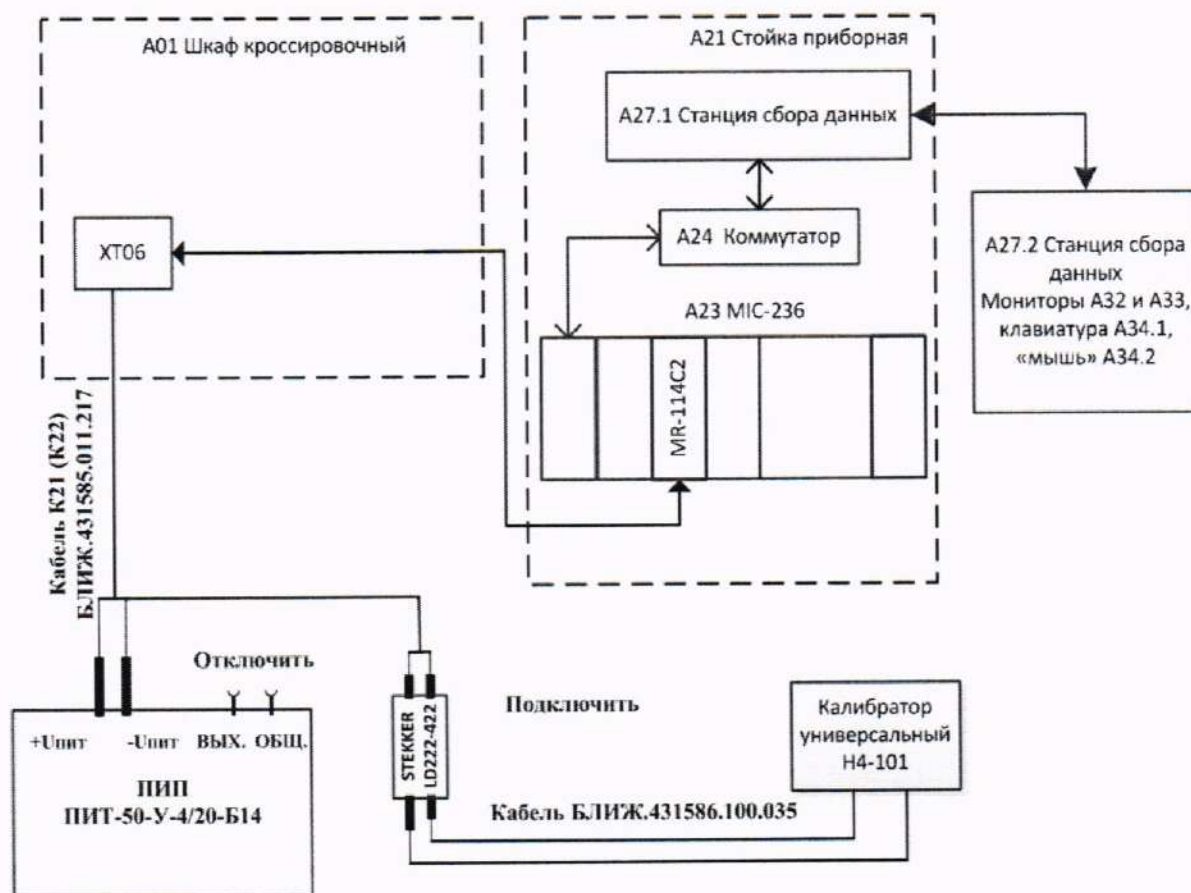
Рисунок 23 – Схема поверки электрических частей ИК силы постоянного тока
