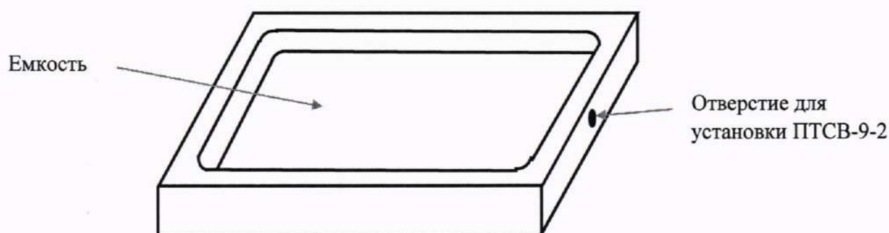
Рисунок А.1 - Схема установки ПТСВ-9-2 в плиту алюминиевую при проверке диапазона и определении погрешности измерений температуры дорожного полотна
