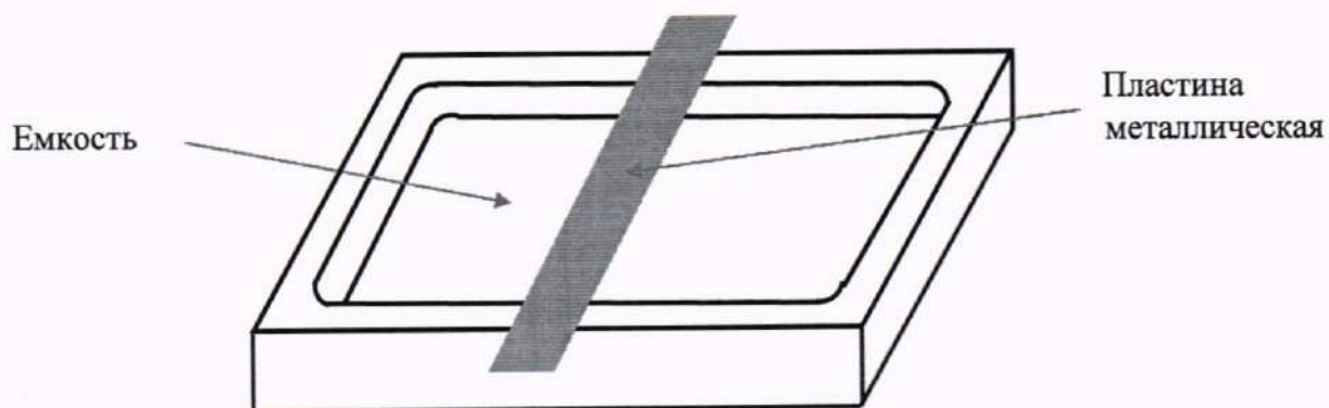
Рисунок В.1 - Схема установки пластины металлической на плиту алюминиевую при проверке диапазона измерений и определении абсолютной погрешности измерений толщины слоя льда
