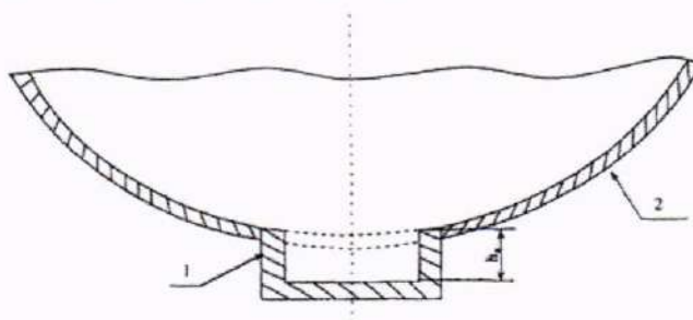
1 – прямик; 2 – цилиндрическая часть танка h_n – высота прямка
