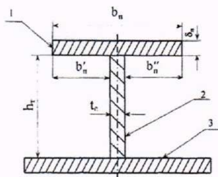
1 – полка профиля; 2 – стенка профиля; 3 – присоединенный пояс обшивки b_n, \delta_n – длина и толщина полки; h_r, t_n – высота и толщина стенки профиля; b'_n, b''_n – расстояние от торцов полки до стенки профиля
