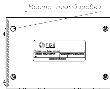
Рисунок 11 – Схема пломбировки для вычислительного устройства ИВБ (КМ-М-6И)
