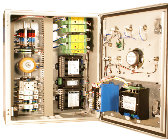
Рисунок 5 – Общий вид шкафа диспетчеризации с голосовой связью (Риталл, 500×400×250 мм) (пример)
