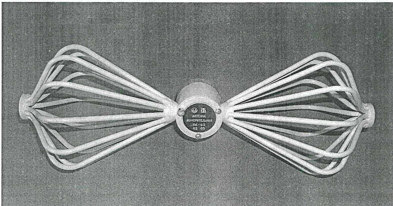
Рисунок 1 - Антенна измерительная П6-62. Внешний вид.
