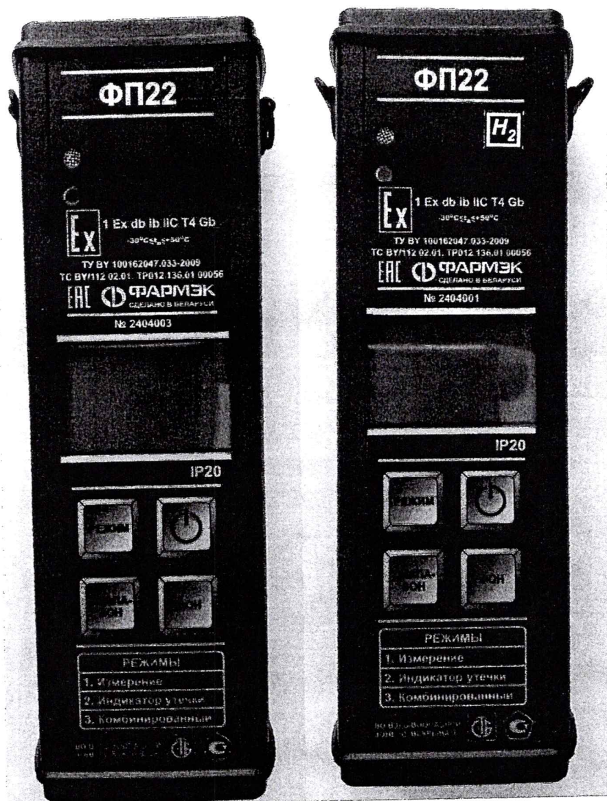
Рисунок 1.1 – Фотографии общего вида и маркировки газоанализаторов ФП22 (изображение носит иллюстративный характер)
