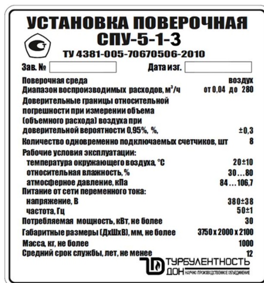
Рисунок 6 – Общий вид маркировочной таблички
