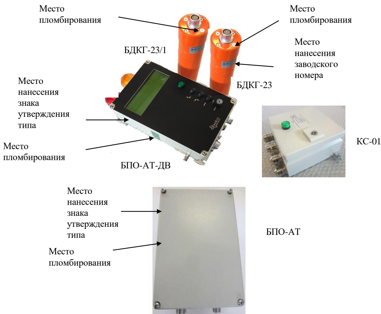
Рисунок 1 – Установка дозиметрическая для измерения мощности дозы гамма-излучения УДМГ-104, обозначение мест пломбирования, место нанесения заводского номера и знака утверждения типа
