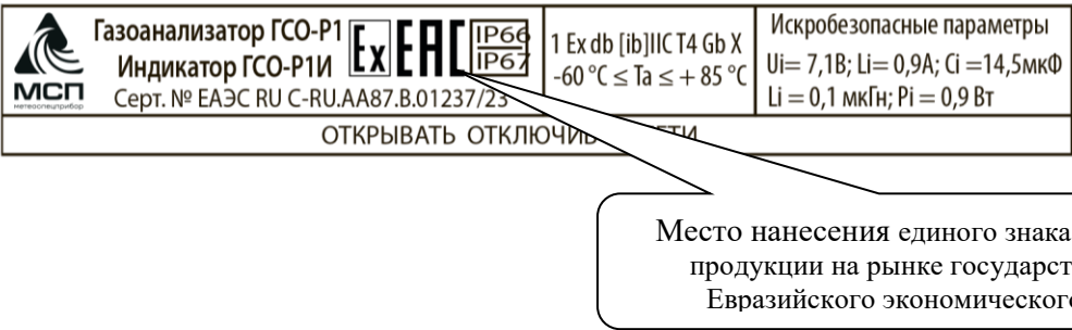
Рисунок 9 – Общий вид таблички, расположенной на корпусе индикатора ГСО-Р1И
