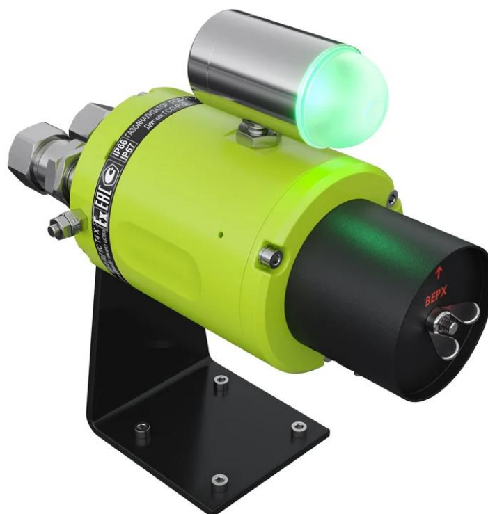
Рисунок 6 – Общий вид газоанализаторов стационарных оптических ГСО-Р1, датчик ГСО-Р1Д со свето-звуковым оповещателем ГСО-Р1-СЗО
