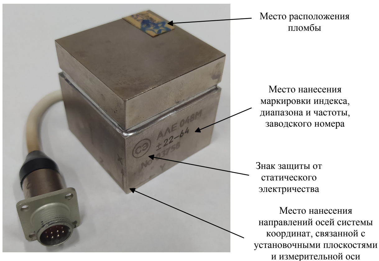
Рисунок 1 – Общий вид акселерометра
