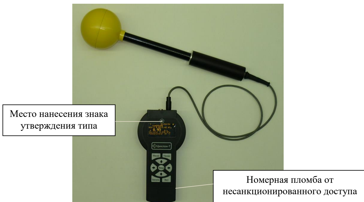
А) Блок измерительный «Циклон-Т» с антенной АЭ1
