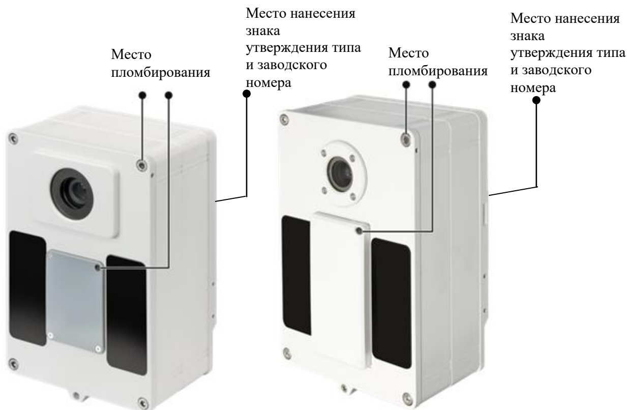
Рисунок 1 – Общий вид, места пломбирования, место нанесения знака утверждения типа и заводского номера комплекса (модификация 1) с квадратной и круглой защитной блендами
